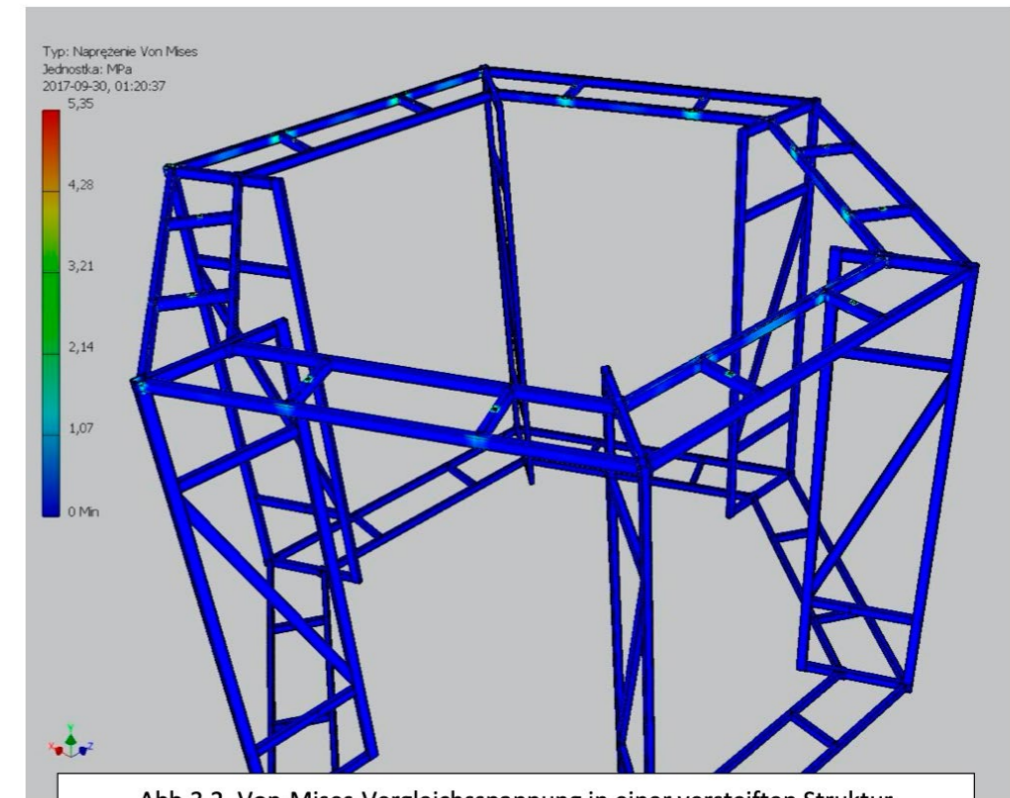
Abb.3.2. Von-Mises-Vergleichsspannung in einer versteiften Struktur
