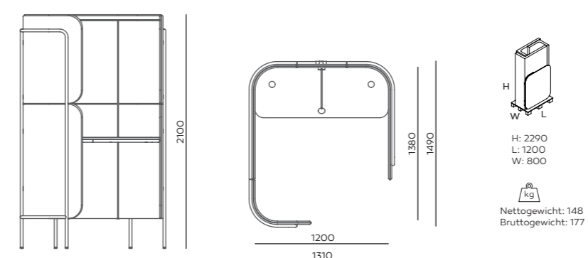
LP STAND H3
